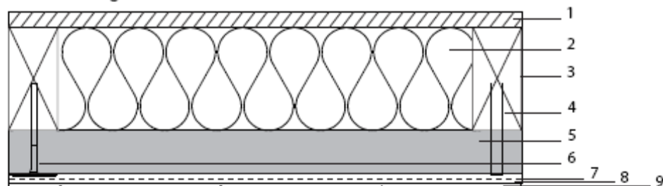
Direkt auf tragende Holzkonstruktion
