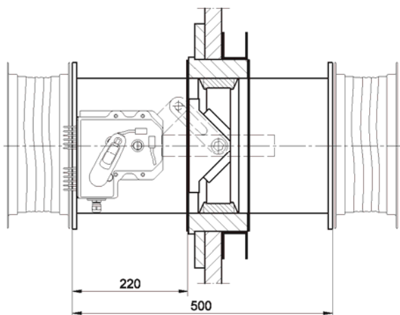
mit Einbaurahmen einseitig bekleidet
