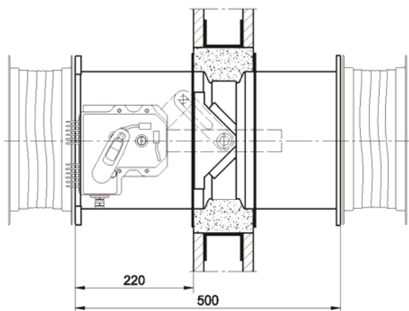
ohne Einbaurahmen im Nasseinbauverfahren
