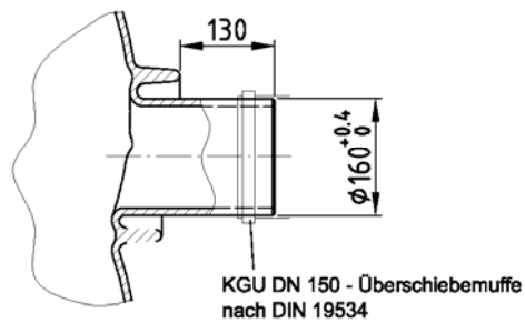
Einzelheit " X " ( Zulauf )
