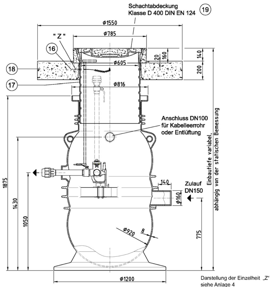
Abb.: Multi-Max-F_Klasse D mit Aufsatzstück
