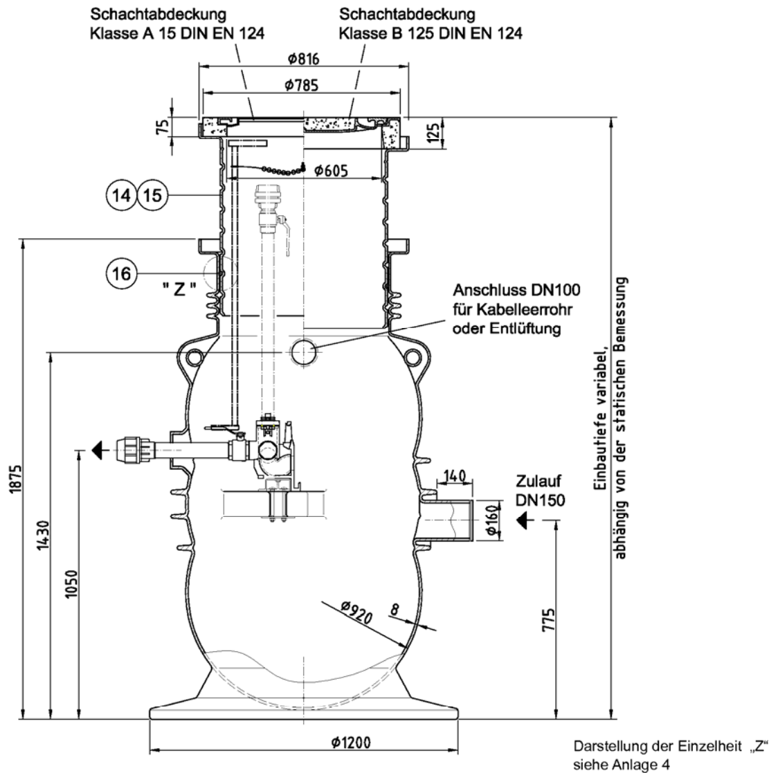
Abb.: Multi-Max-F_Klasse A+B mit Aufsatzstück
