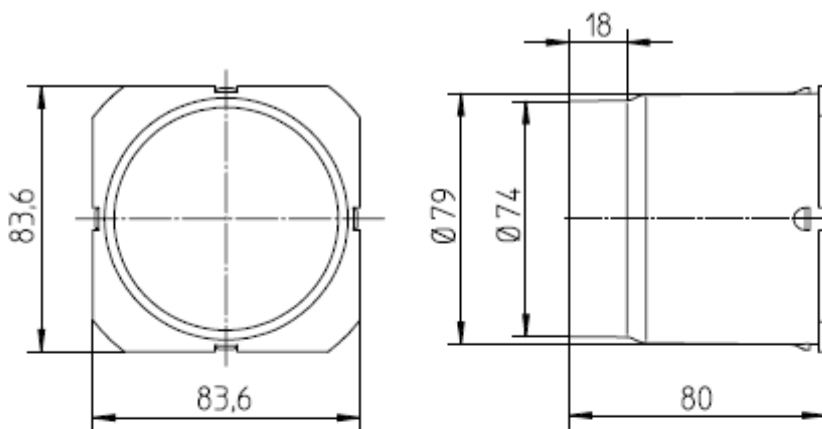
Ausblasstutzen Pos. 14
