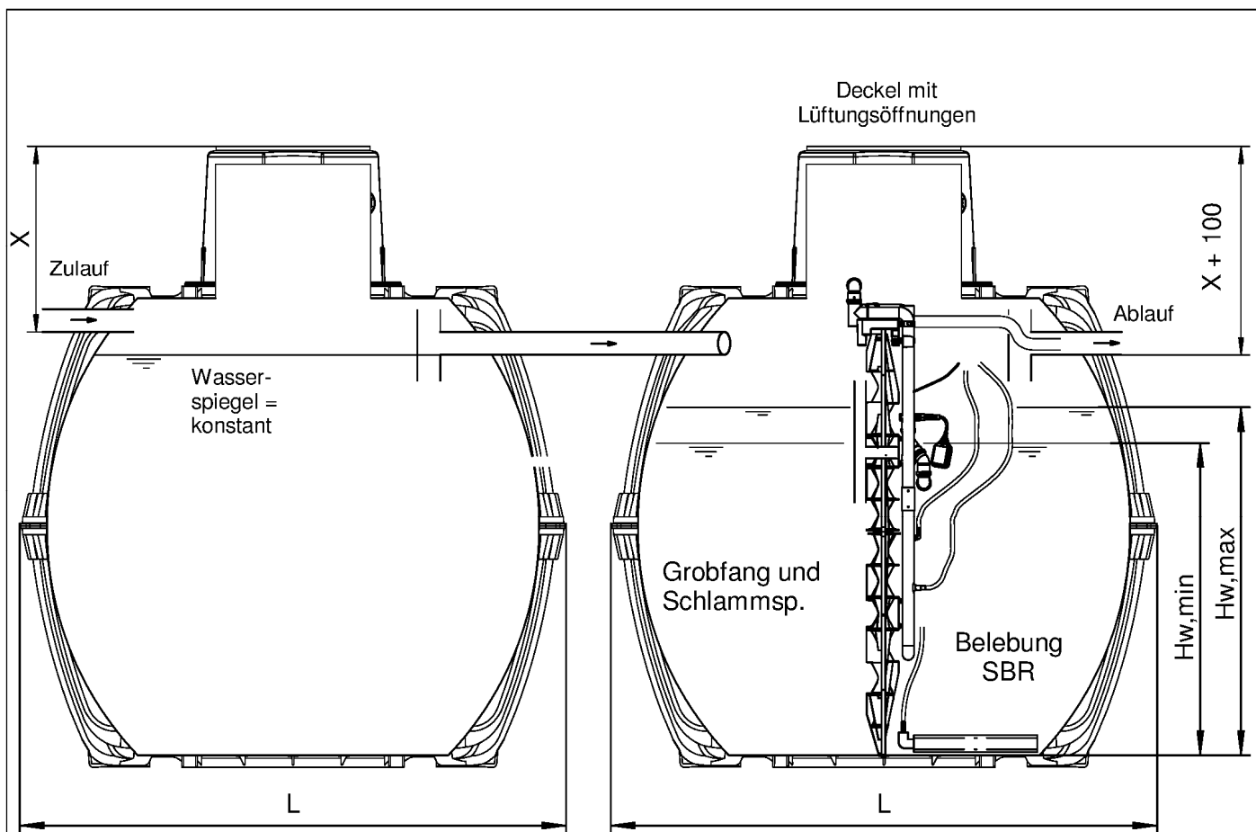
Grobfang und Schlamm Speicher
