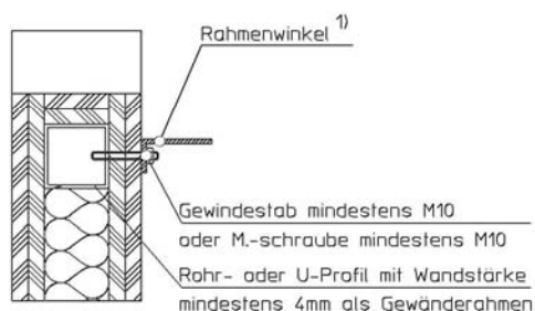
Befestigungsart Nr. 4
