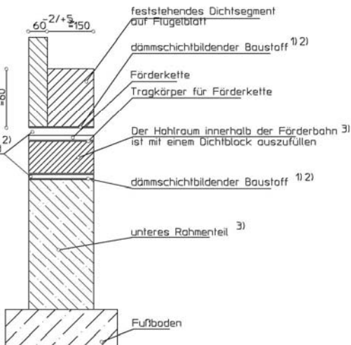
Schnitt A-A
