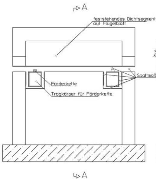
Vorderansicht Kettenfördereranlage (einflügelige Ausführung)
