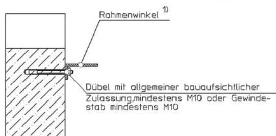
Befestigungsart Nr. 2 Dübel mit allgemeiner bauaufsichtlicher Zulassung
