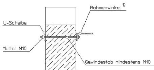
Befestigungsart Nr. 1 durchgehender Gewindestab
