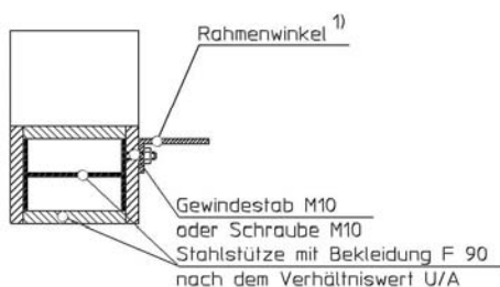
Befestigungsart Nr. 3
