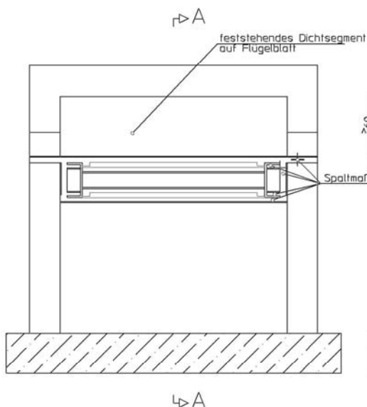
Vorderansicht Gurtfördereranlage (einflügelige Ausführung)
