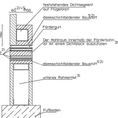
Schnitt A-A
