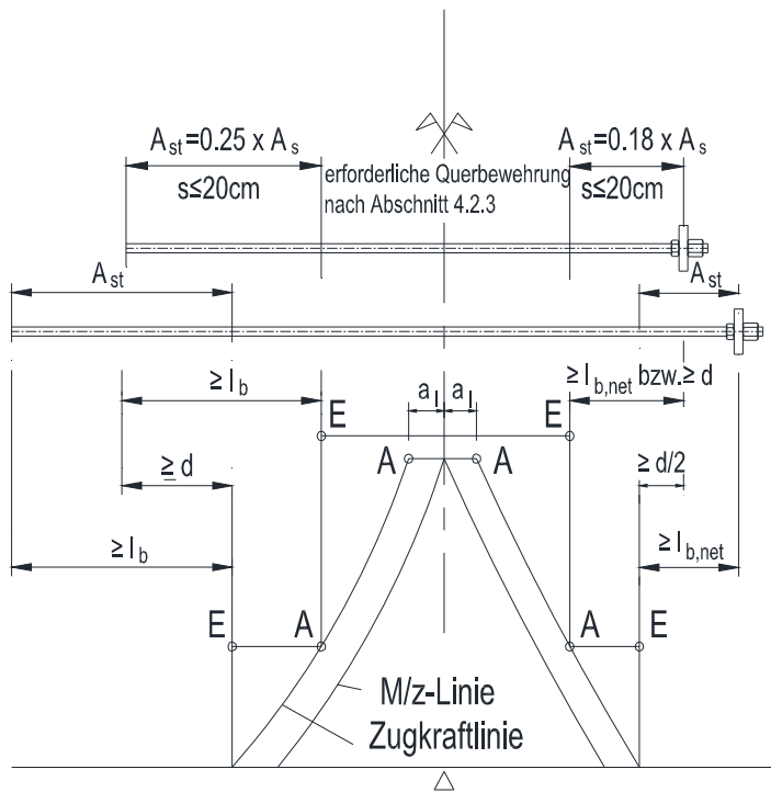
Bild 3b: Beispiel für die Verankerung von Stäben d_s = 40 bis 50 mm mit geraden Stabenden und Ankerplatten im Stützbereich massiger Bauteile nach Abschnitt 4.2.2
