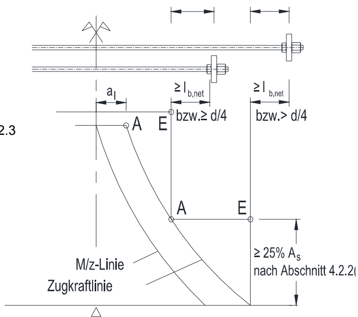
Bild 3b: Beispiel für die Verankerung von Stäben d_s = 40 bis 50 mm mit geraden Stabenden und Ankerplatten im Stützbereich massiger Bauteile nach Abschnitt 4.2.2
