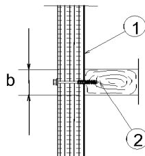
Bild 2 Holzaufleger
