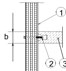
Bild 3 Betonaufleger
