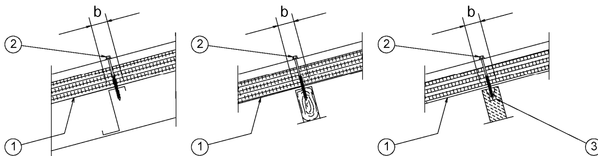
Bild 1 Stahlaufleger
