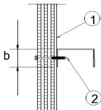
Bild 1 Stahlaufleger
