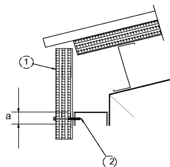
Bild 6 Traufpunkt
