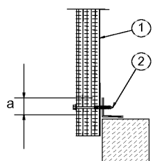
Bild 5 Fusspunkt Wandelement vorgehängt
