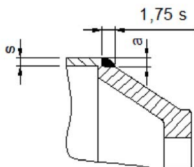
Überlappnaht
