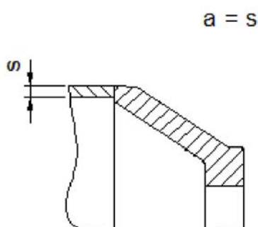
Lasernaht, I-Naht
