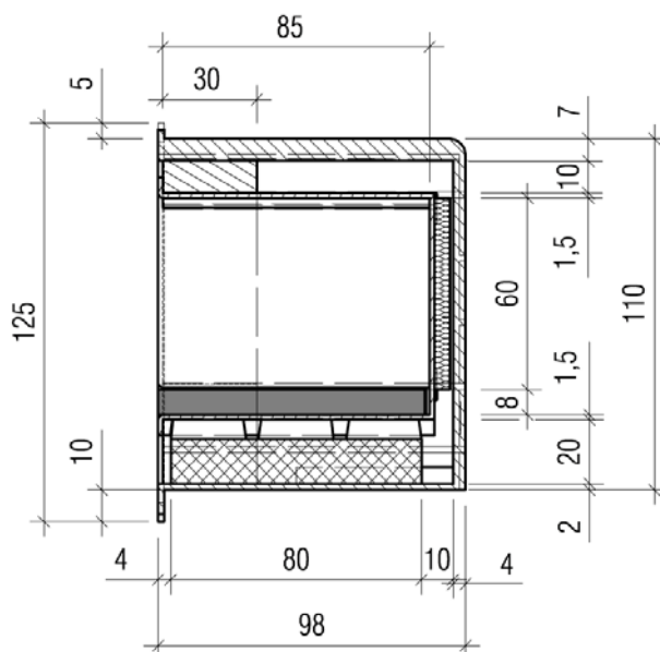
Vertikalschnitt:
