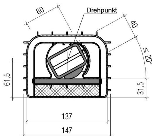
Drehwinkel ± 20° (Einbau im Treppenlauf)
