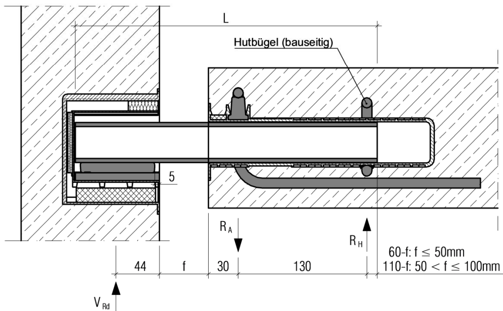
Statisches System
