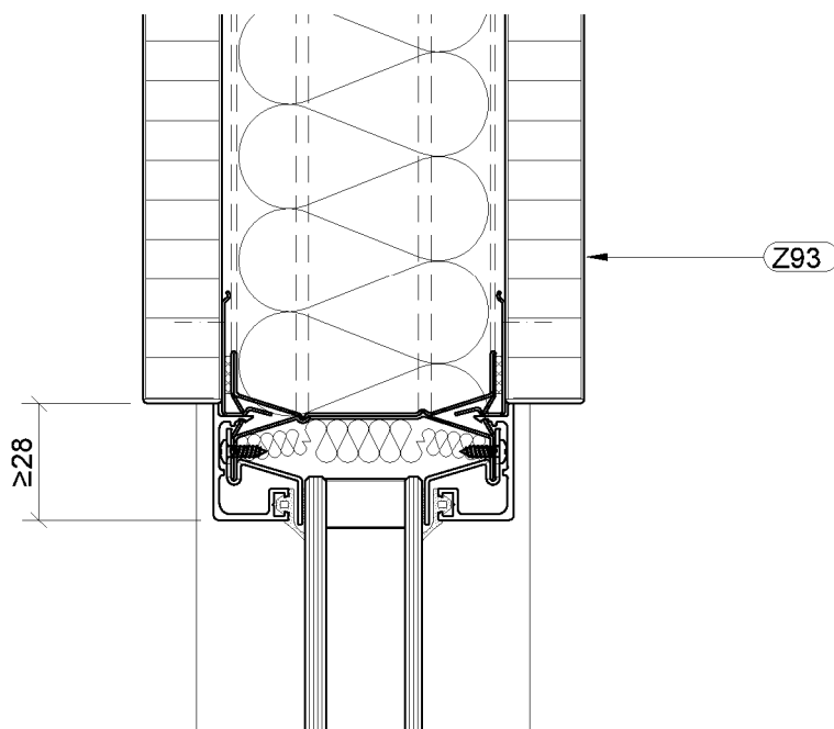
Schnitt E-E/4 Querfuge Glas / Vollwand mit Halbriegel
