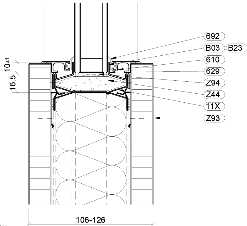
Schnitt E-E/1 Querfuge Vollwand / Glas verdeckter Anschluss
