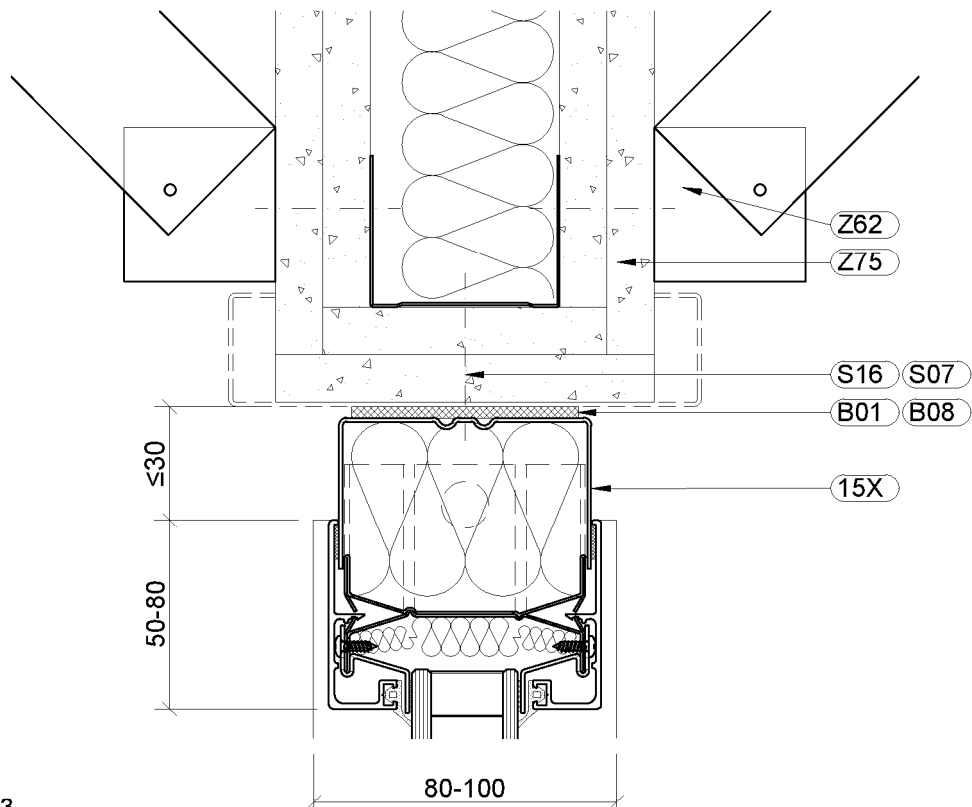
Schnitt D-D/3 Anschluss an Trennwandschürze mit beidseitiger Aussteifung
