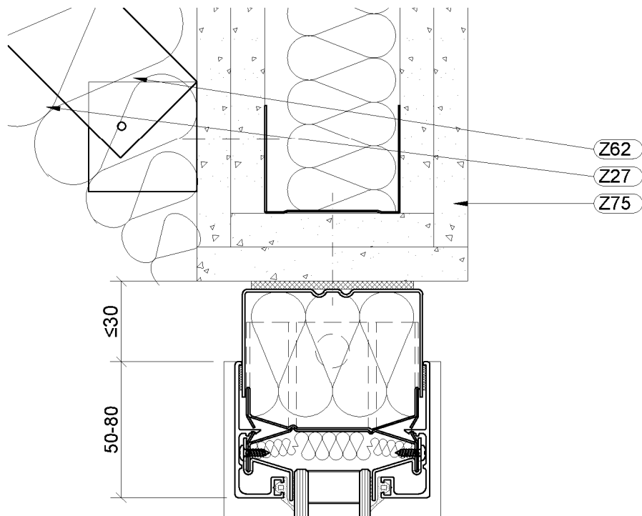
Schnitt D-D/4 Anschluss an Trennwandschürze mit einseitiger Aussteifung
