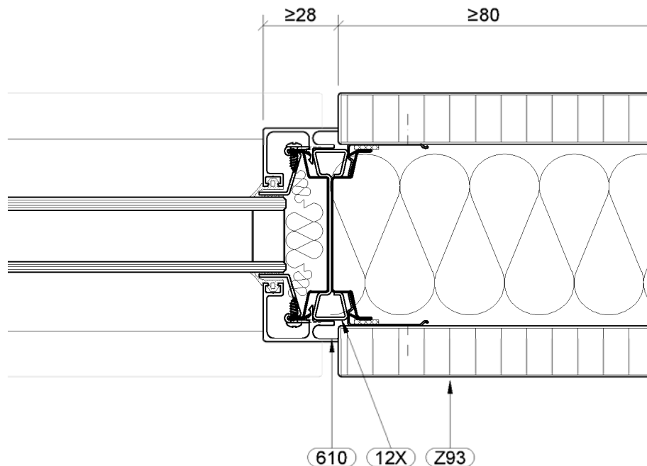
Schnitt B-B/2 Systemanschluss mit Regalständer
