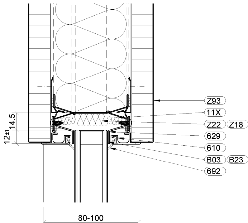
Schnitt E-E/3 Querfuge Glas / Vollwand verdeckter Anschluss
