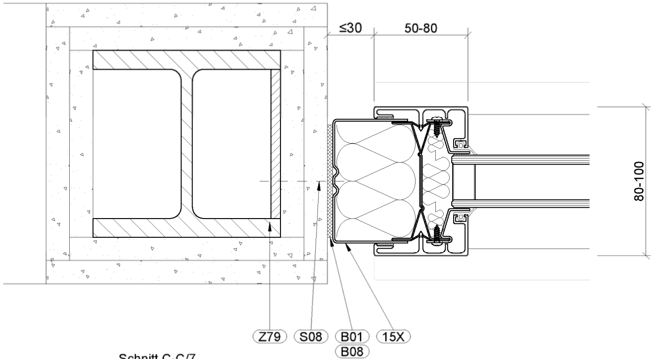
Schnitt C-C/7 Anschluss an bekleidete Stahlstütze
