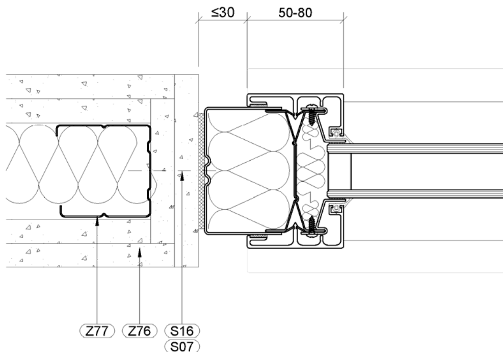
Schnitt C-C/6 Anschluss an GK-Wand, längs
