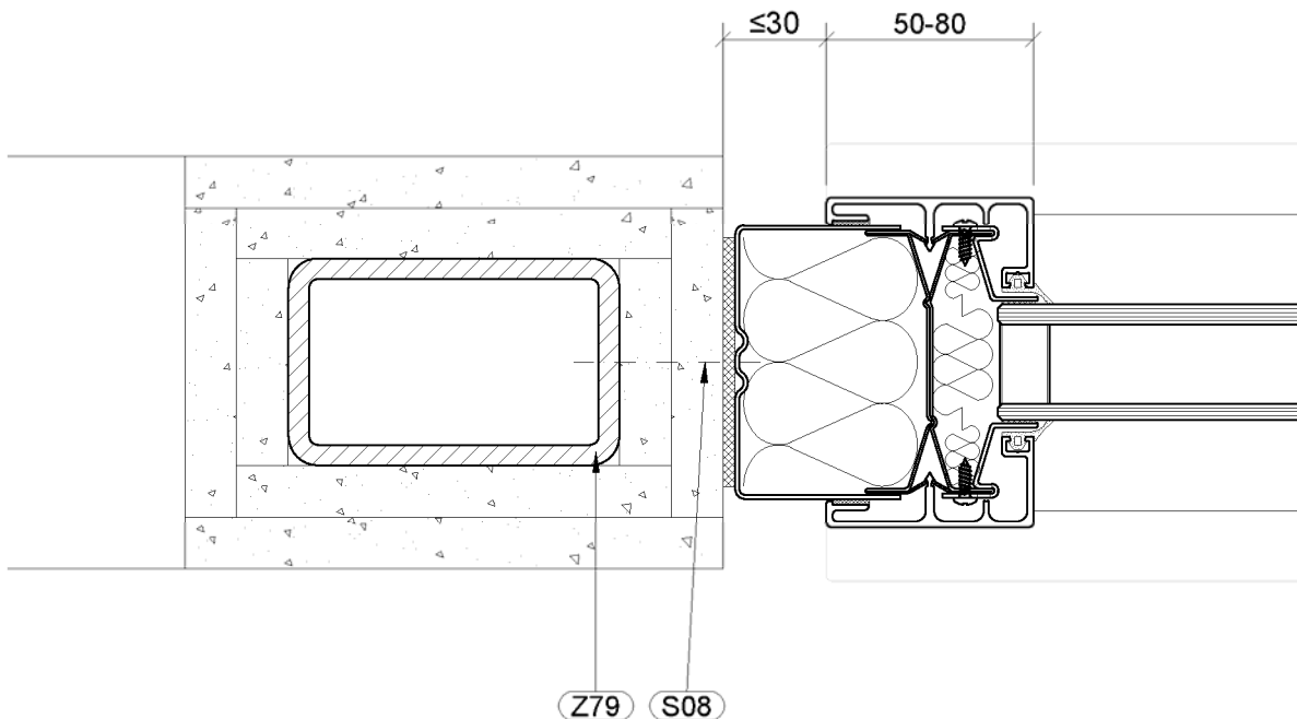
Schnitt C-C/8 Anschluss an bekleidete Stahlstütze
