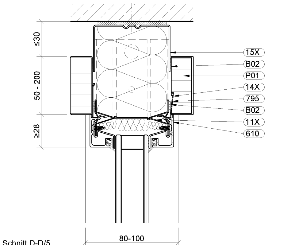
Schnitt D-D/5 Deckenanschluss mit Blende
