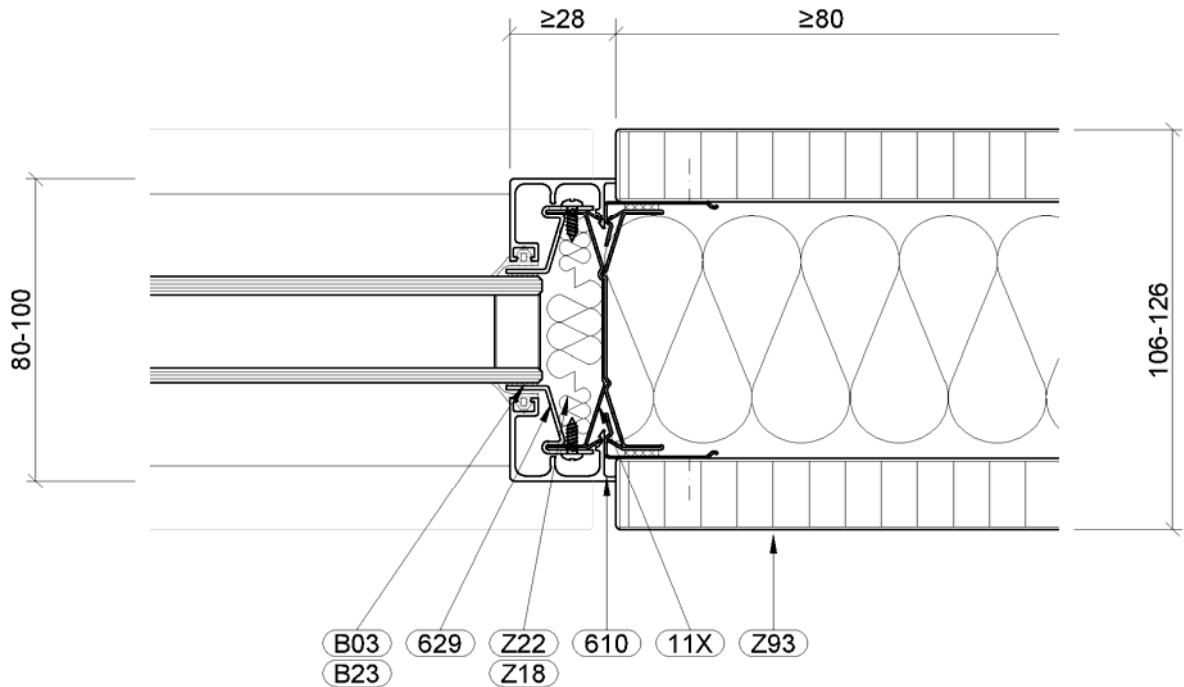
Schnitt B-B/1 Systemanschluss an feco-Vollwand F30
