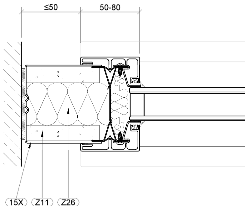
Schnitt C-C/2 Wandanschluss mit großer Fuge
