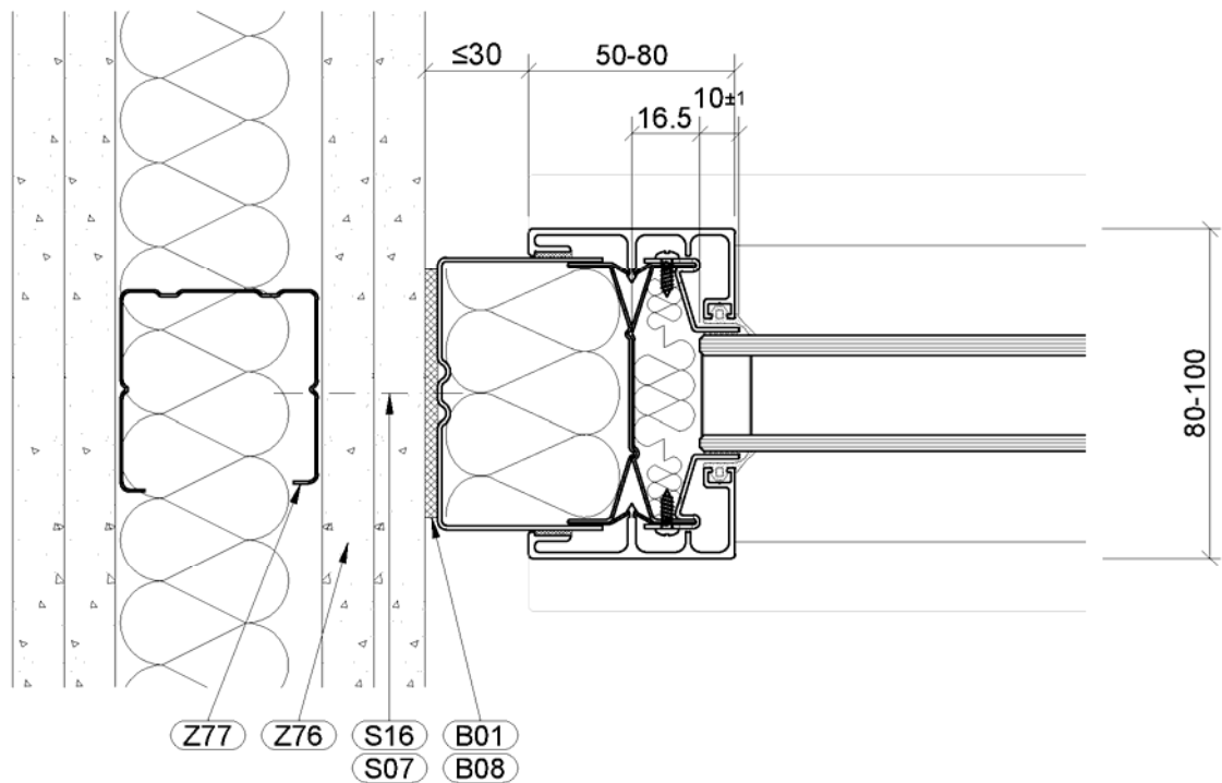
Schnitt C-C/5 Anschluss an GK-Wand, quer
