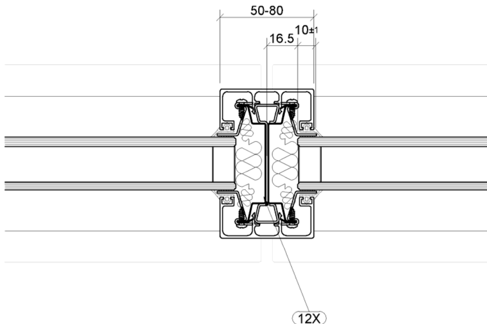
Schnitt A-A/2 Mittelfuge mit Regalstander
