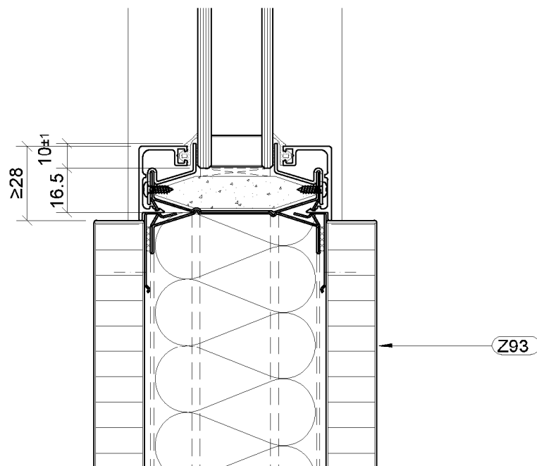
Schnitt E-E/2 Querfuge Vollwand / Glas mit Halbriegel
