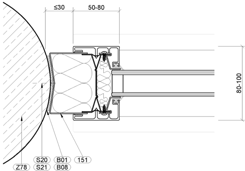
Schnitt C-C/9 Anschluss an Rundstütze
