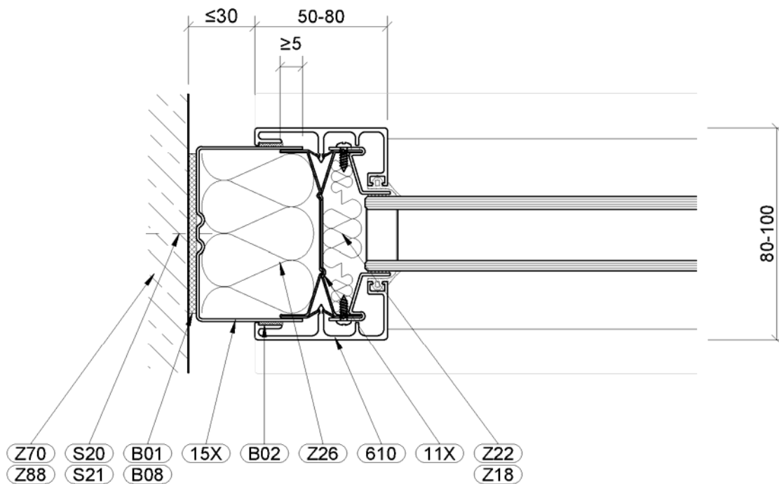
Schnitt C-C/1 Wandanschluss
