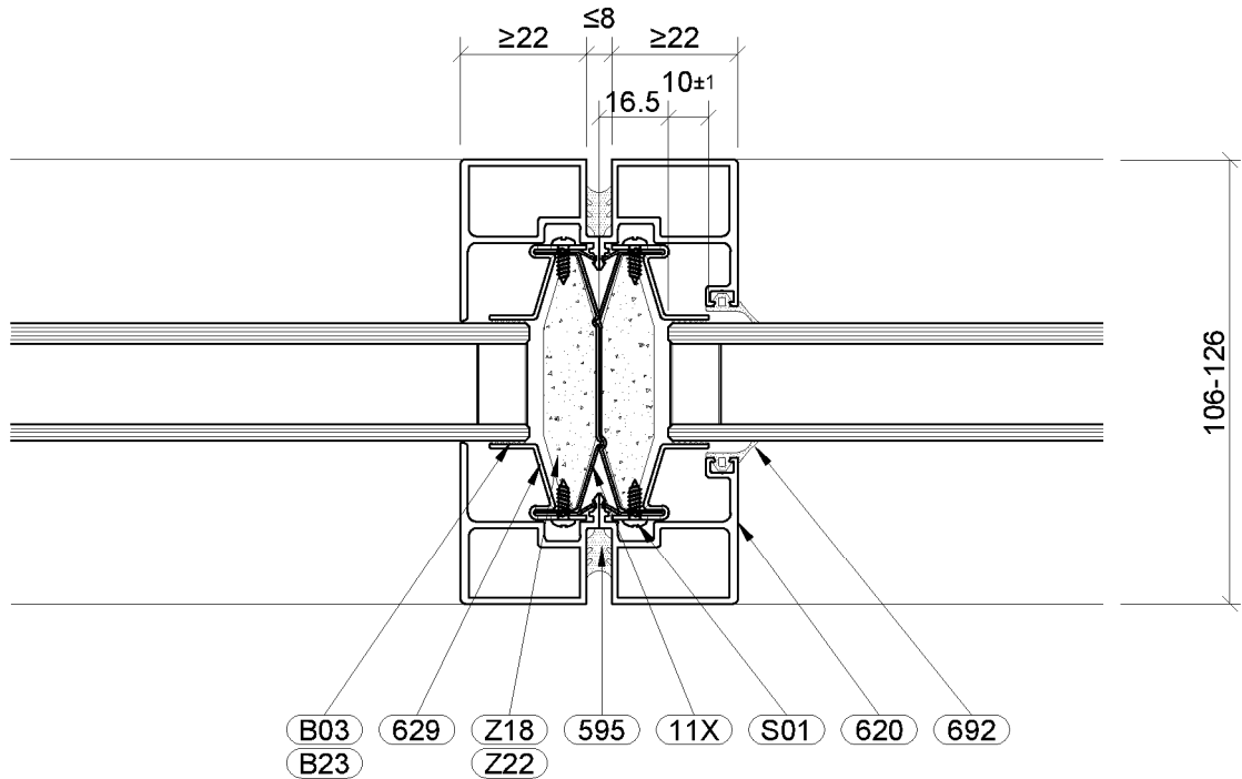
Schnitt A-A/3 Mittelfuge mit Abdeckrahmen
