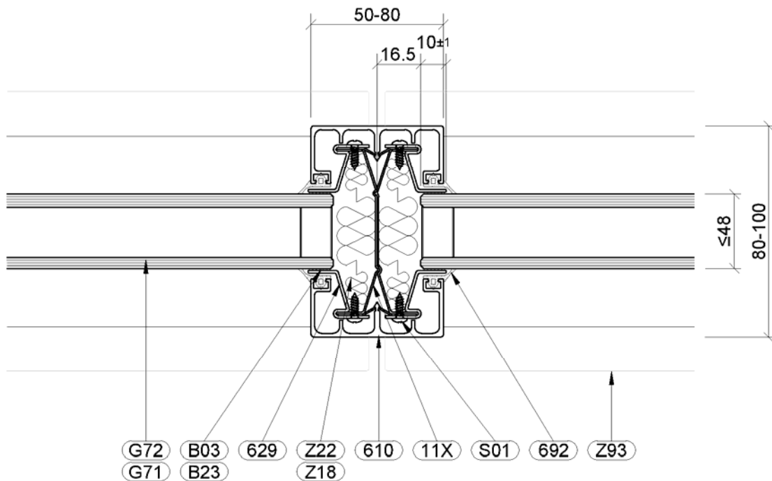
Schnitt A-A/1 Mittelfuge mit Normalständer
