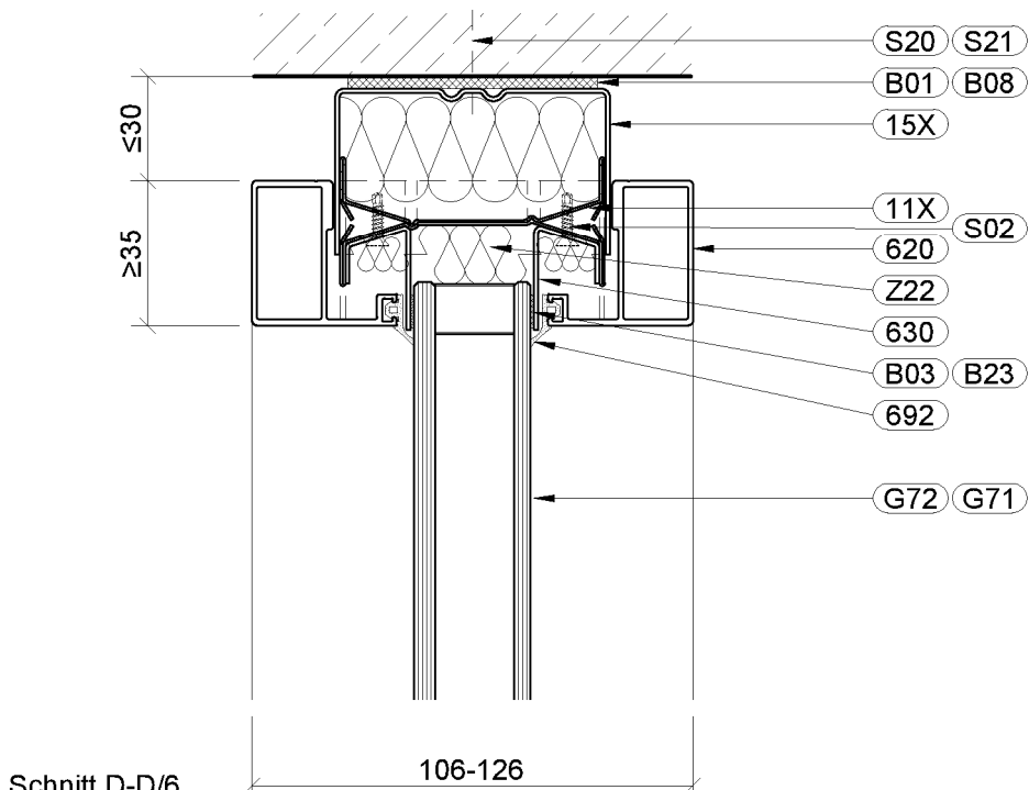
Schnitt D-D/6 Deckenanschluss mit Abdeckrahmen
