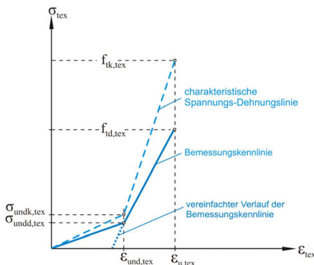
Bild abZ 5.1: Idealisierte Spannungs-Dehnungslinie für Textilbeton
