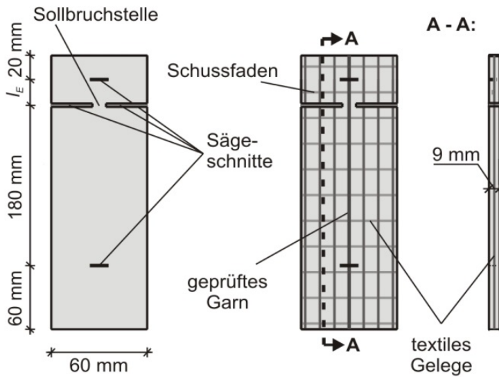
Bild 4: Probekörperaufbau für den Textilauszugsversuch
