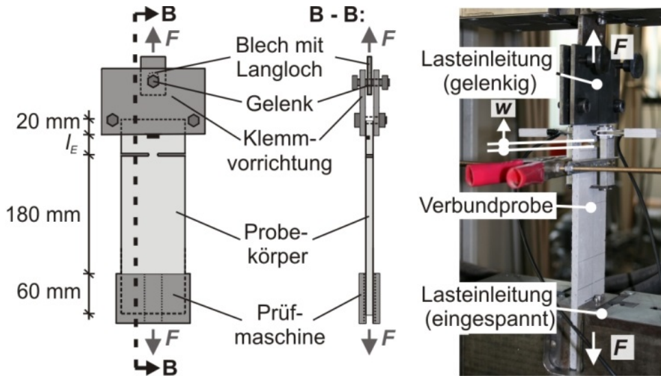
Bild 5: Versuchsaufbau des Textilauszugsversuchs
