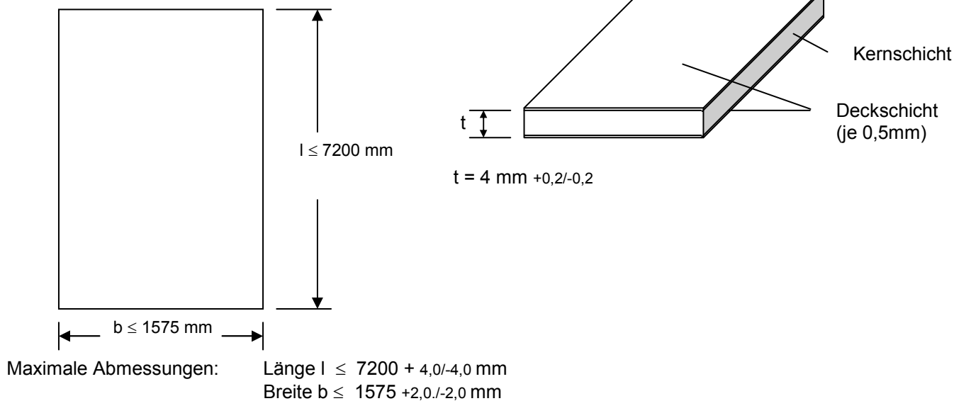
Fassadenplatte nach Abschnitt 2.2.1
