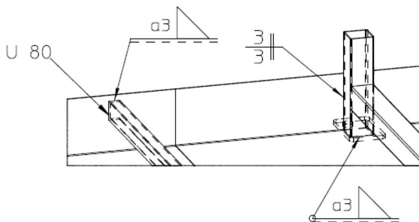
Detail 2 Mittelstütze
