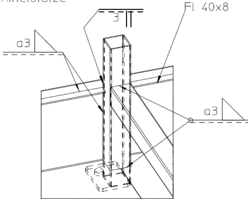
Detail Mittelstütze
