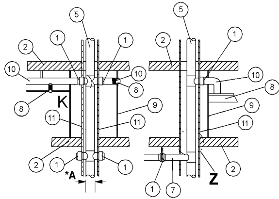
Einbaubeispiel Zentrallüftungsanlage
