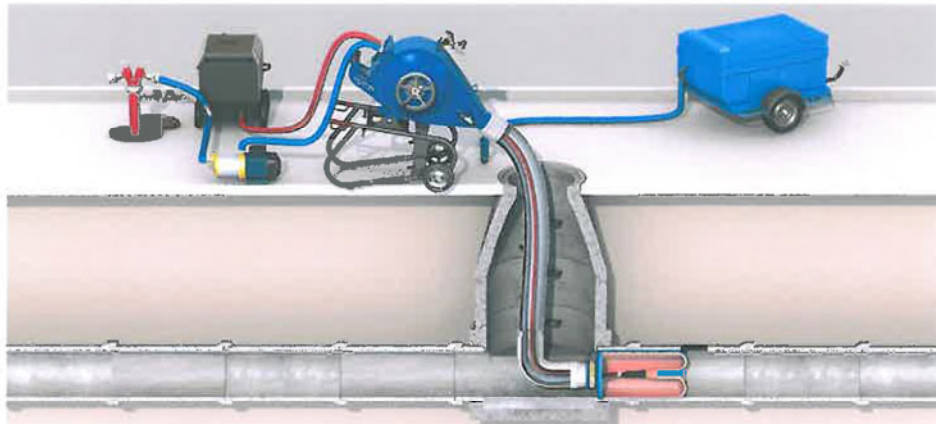
1. Schlauchliner mit Kalibrierschlauch am Startpunkt positionieren.
