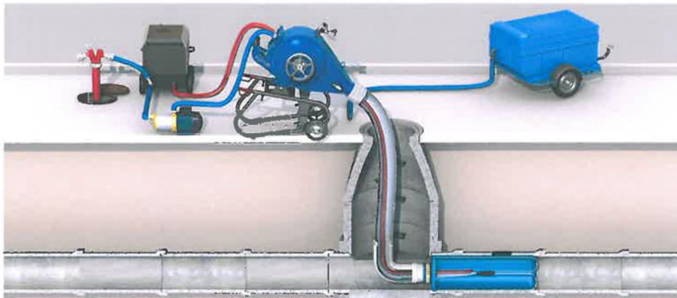
2. Inversion des Schlauchliners, Heizschlauch wird mit inversiert.
