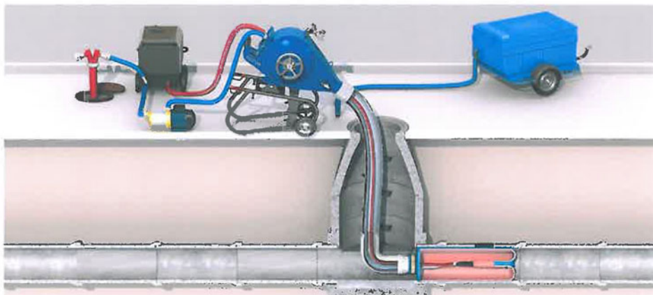
2. Schlauchliner mit Kalibrierschlauch gleichzeitig invertieren.
