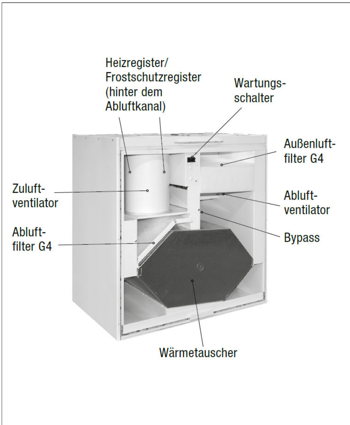
Zentrales Lüftungsgerät mit Wärmerückgewinnung Typ "VALLOX ValloPlus 350 SE"
