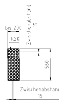
Detail Koaleszenzgitter
