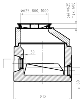
Probenmeschacht als Probenahmevorrichtung gemäß DIN 1999-100
