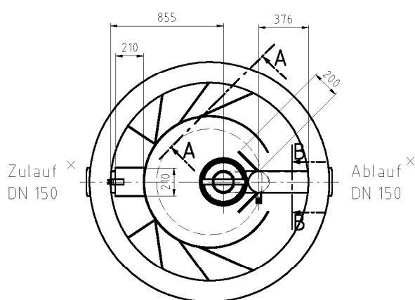
Detail Zulaufprallblech
