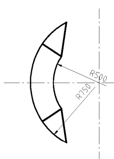
Detail Zulaufprallblech
