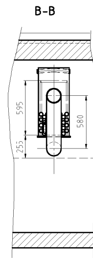
Detail Koaleszenzgitter
