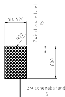
Detail Koaleszenzgitter
