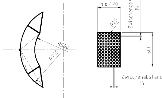
Detail Zulaufprallblech
