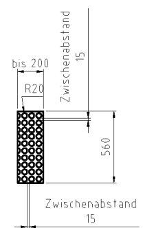
Detail Koaleszenzgitter
