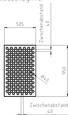
A-A Detail Koaleszenzgitter
