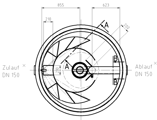
Detail Zulaufprallblech
