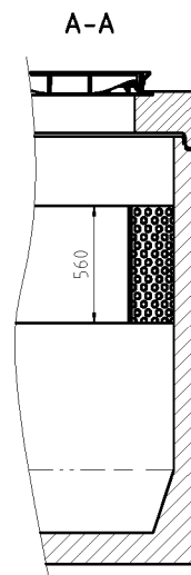
Detail Bodenplatte Koaleszenzkanal
