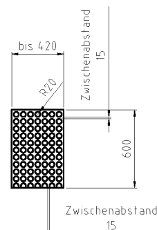
Detail Koaleszenzgitter
