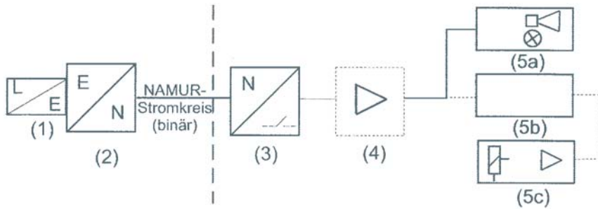
Schema der Überfüllsicherung
