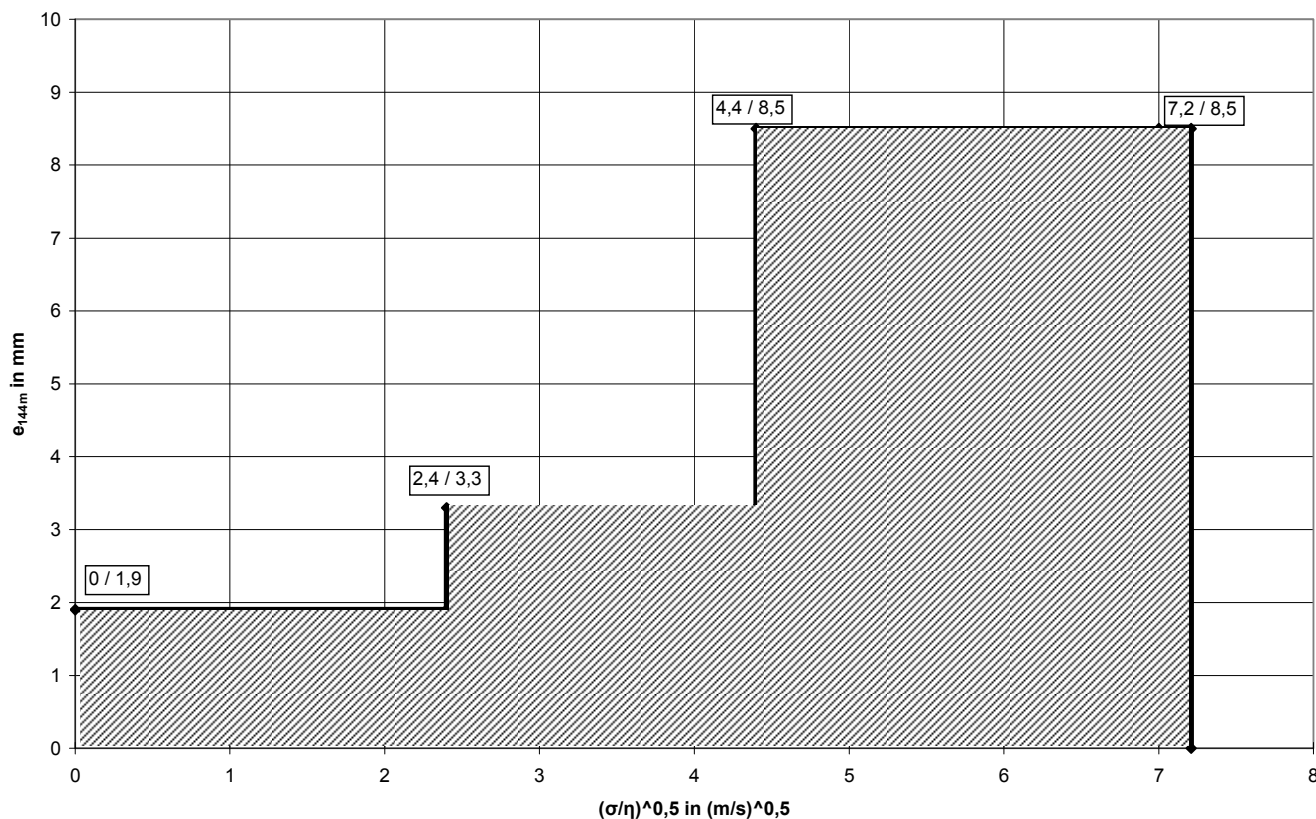
Abbildung 1: Eindringverhalten (mittlere Eindringtiefe e_{144\text{m}} von Flüssigkeiten) 1) , aufgrund der jeweiligen dynamischen Viskosität und Oberflächenspannung.
