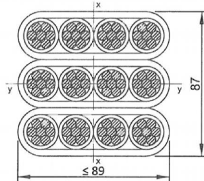
VBT-BE 3x4-150
