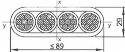
VBT-BE 4-150
