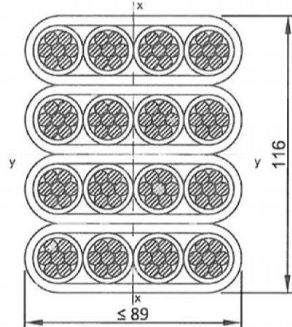
VBT-BE 4x4-150
