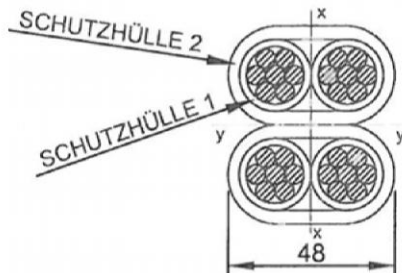
VBT-BE 2x2-150
