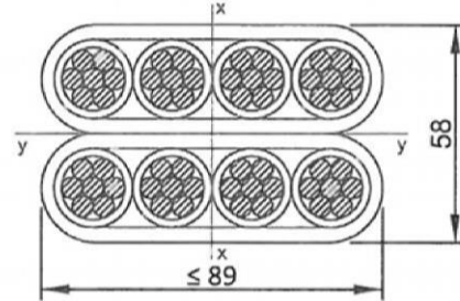
VBT-BE 2x4-150
