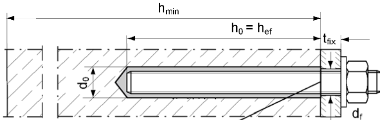
Ankerstange Vorsteckmontage
