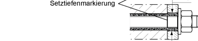
Ankerstange Durchsteckmontage (Ringspalt mit Mörtel verfüllt)
