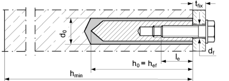
fischer Innengewindeanker RG MI Nur Vorsteckmontage
