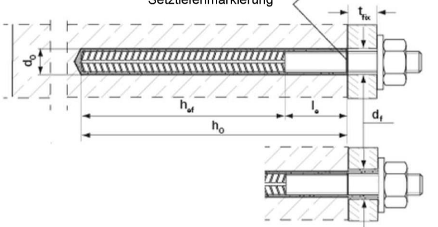
Bewehrungsanker BRA Durchsteckmontage (Ringspalt mit Mörtel verfüllt)
