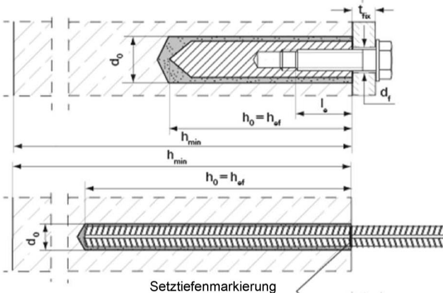
Innengewindeanker MCS Plus I nur Vorsteckmontage
