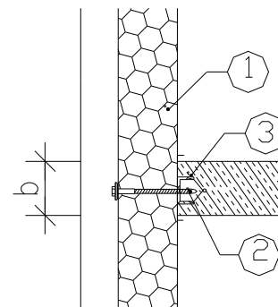
Bild 3 Betonaufleger
