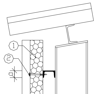
Bild 6 Traufpunkt
