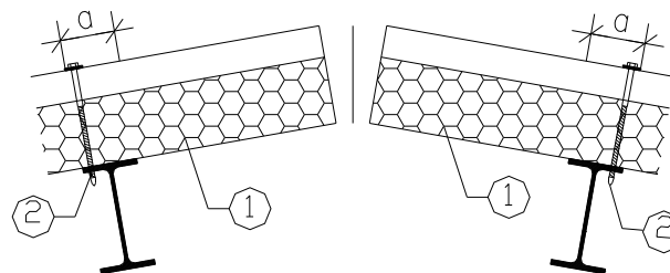
Bild 5 Firstpunkt
