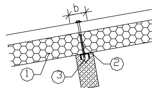
Bild 3 Betonaufleger
