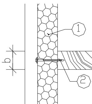
Bild 2 Holzaufleger
