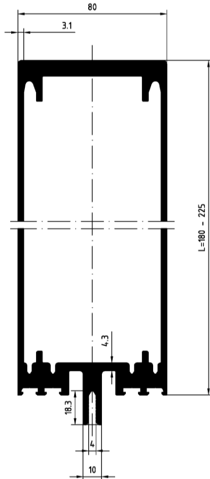
Pfosten
