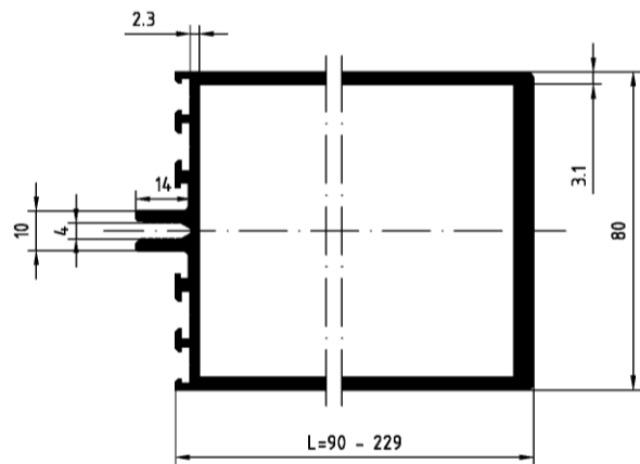
Riegel 1. Ebene
