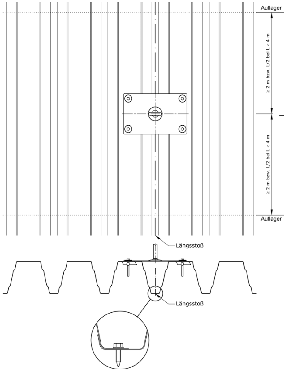
Abbildung 1 – Montagevorgaben auf Trapezprofil (Positivlage)
