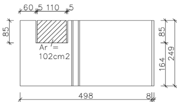
Ansicht Eckstein
