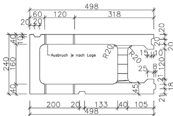
Draufsicht Eckstein
