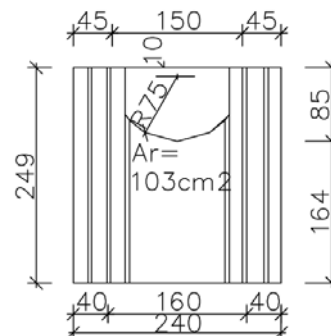
Seitenansicht Eckstein
