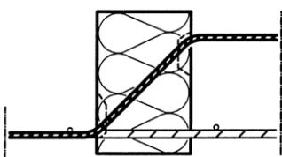
Typ IPTQ/IPTQS
