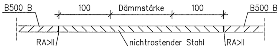
Zugstabvariante 1
