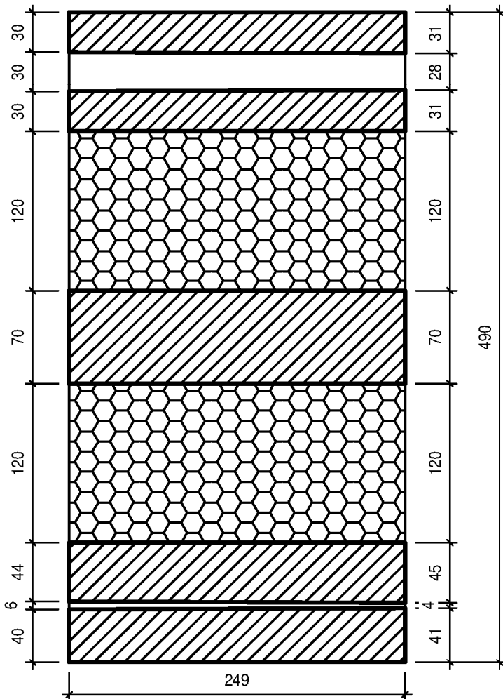
Schnitt B-B
