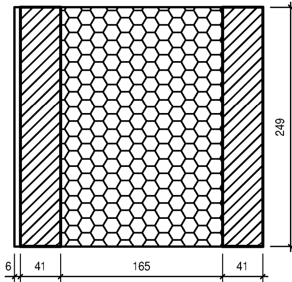
Schnitt B-B
