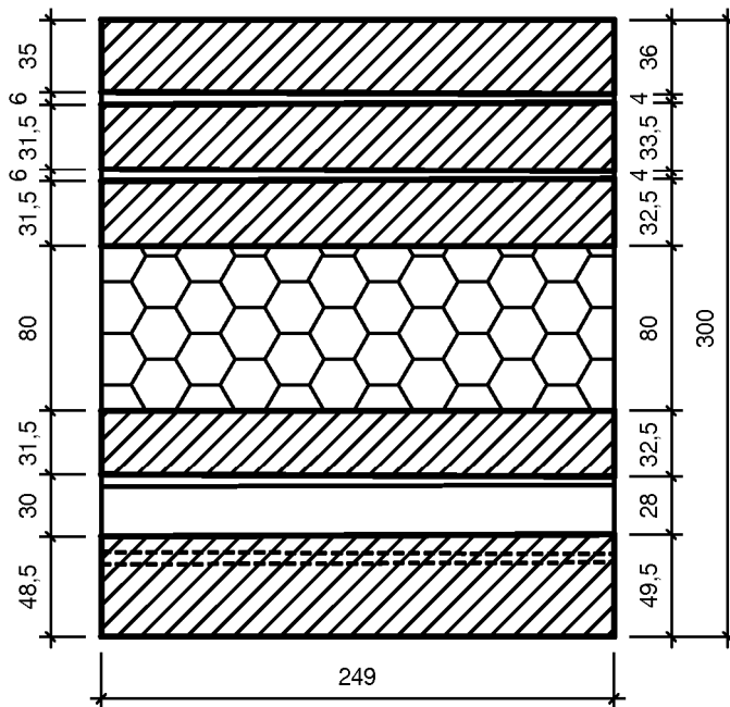
Schnitt B-B
