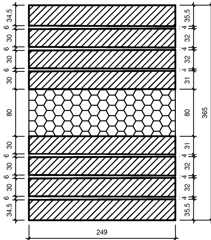
Schnitt B-B
