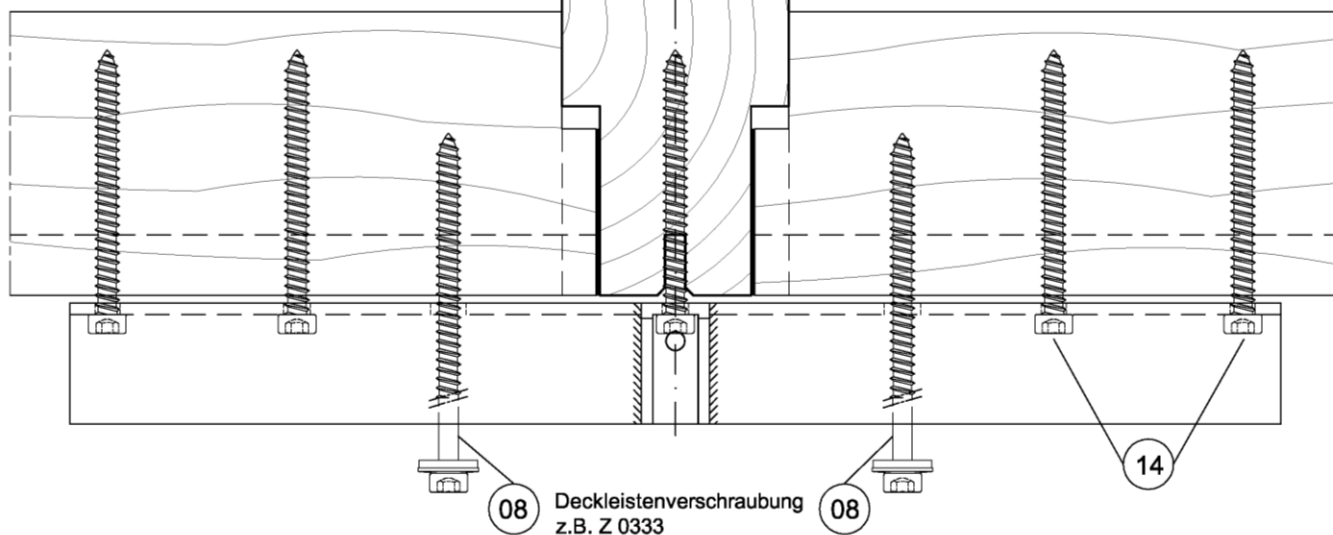
Schnitt G-G
