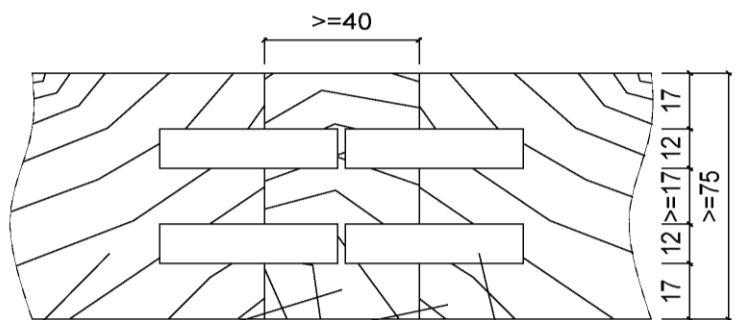
Schnitt F-F
