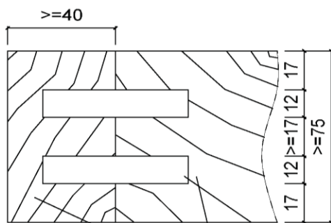
Schnitt E-E
