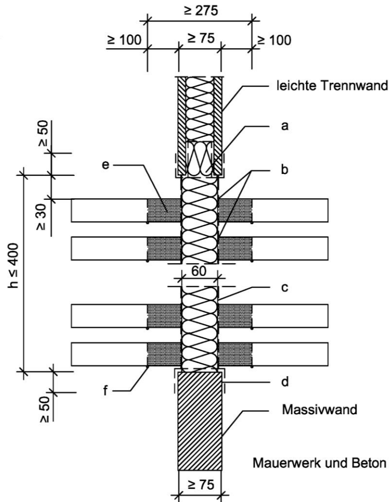
Schnitt B-B
