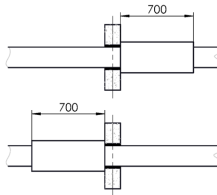
Brandschutzblock stirnseitig an die Wand angrenzend
