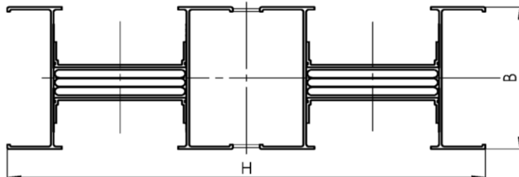
Doppelement Stromschiene "LXA" oder "LXC"
