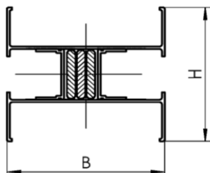
Einfachelement Stromschiene "LXA" oder "LXC"
