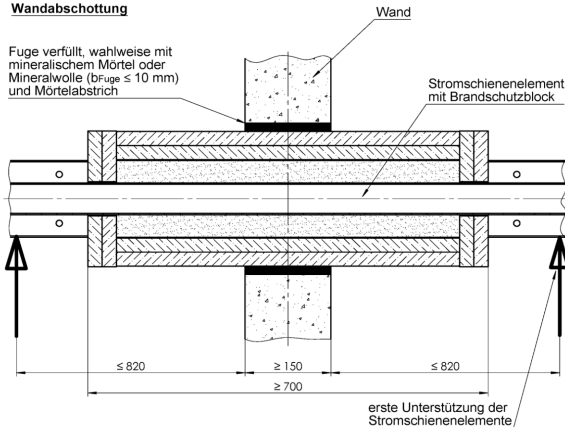
Brandschutzblock in der Rohbauöffnung
