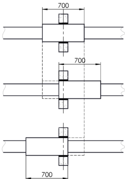
Brandschutzblock in der Rohbauöffnung
