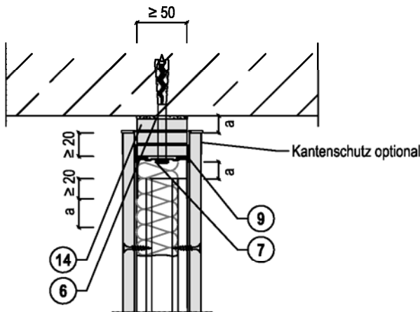
Gleitender Deckenanschluss
