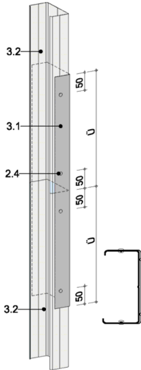
Profilverlängerung Variante 1 Rigips Wandprofile CW ≥ 50 Stumpf gestoßen und zusätzlich mit einem Rigips Wandprofil UW ≥ 50 verbunden
