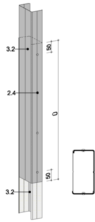
Profilverlängerung Variante 3 Rigips Wandprofile CW ≥ 50 mit einem Rigips Wandprofil CW ≥ 50 zum "Kastenprofil" verbunden
