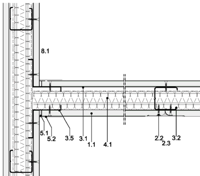
T-Anschluss an eine durchgehende Trennwand mit ausgesparter Beplankung Variante 4
