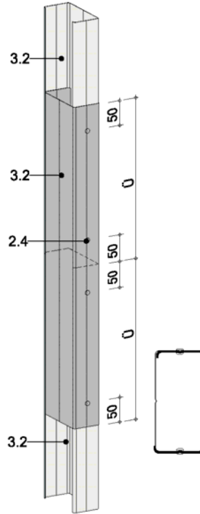
Profilverlängerung Variante 2 Rigips Wandprofile CW ≥ 50 Stumpf gestoßen und zusätzlich mit einem Rigips Wandprofil CW ≥ 50 verbunden
