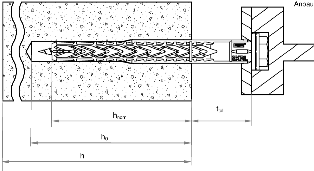
Bild 1: Dübel im Einbauzustand
