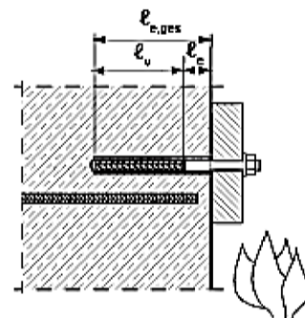
Upat Bewehrungsanker
