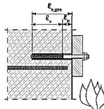
Bewehrungsanker FRA
