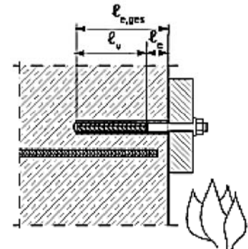
Bewehrungsanker FRA
