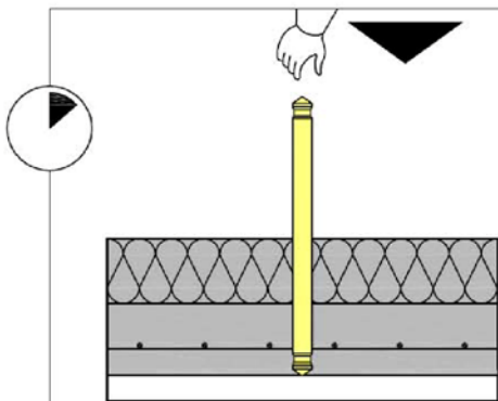
Spätestens 60 Minuten nach Zugabe des Anmachwassers Syspro-Perfect-Verbindungsstäbe bis zum Anschlag am Schalboden in den Frischbeton einsetzen.
