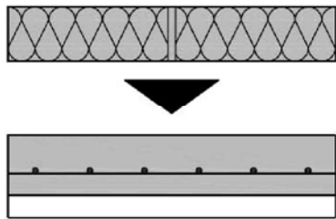
Vorgebohrte Dämmplatten auf dem frischen Beton der Vorsatzschale verlegen.
