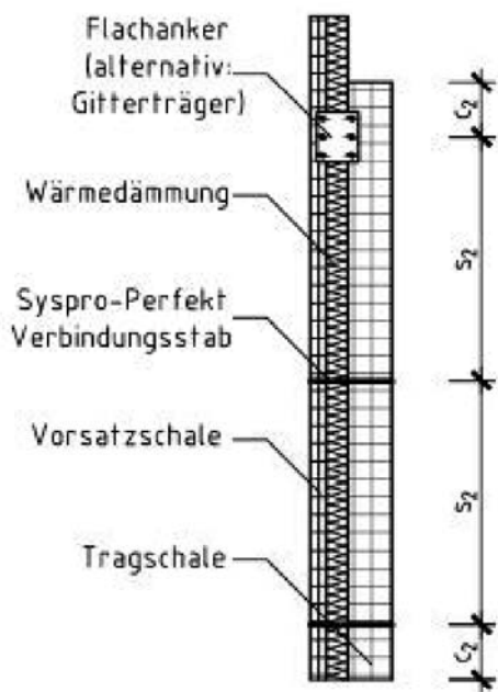
Schnitt A-A Sandwichwand
