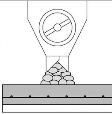
Beton der Vorsatzschale einfüllen und verdichten.
