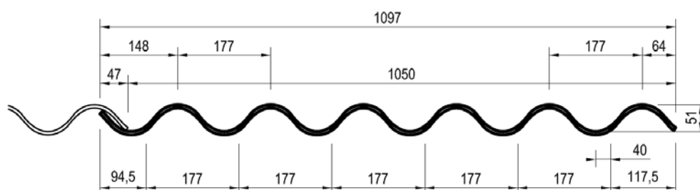
Bild 2: P6 mit 6 Wellen
