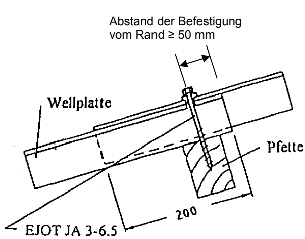
Bild 4a: Anordnung der Befestigung auf Holzpfetten
