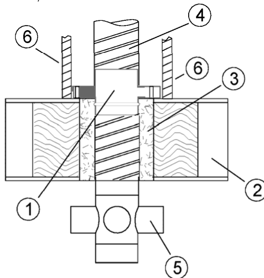
Einbau auf der Geschossdecke aus Holz, Holzbalkendecke F 30-B
