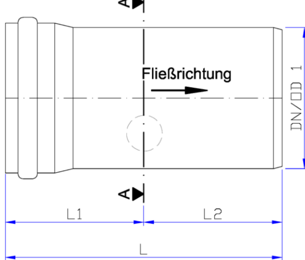
Vorderansicht
