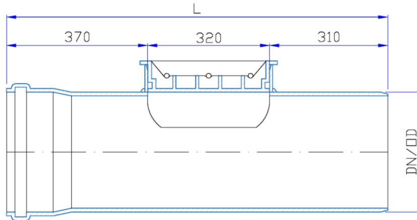
Schnitt A-A
