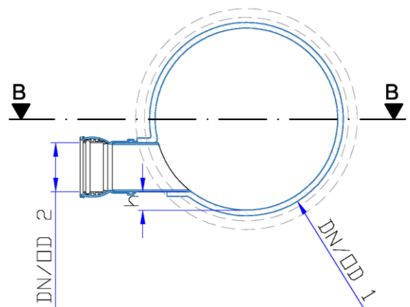
Schnitt A-A
