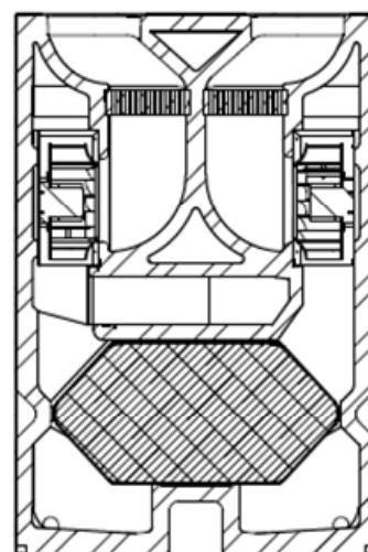
Schnitt A - A
