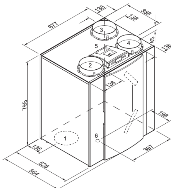
Rechtausführung 3/1
