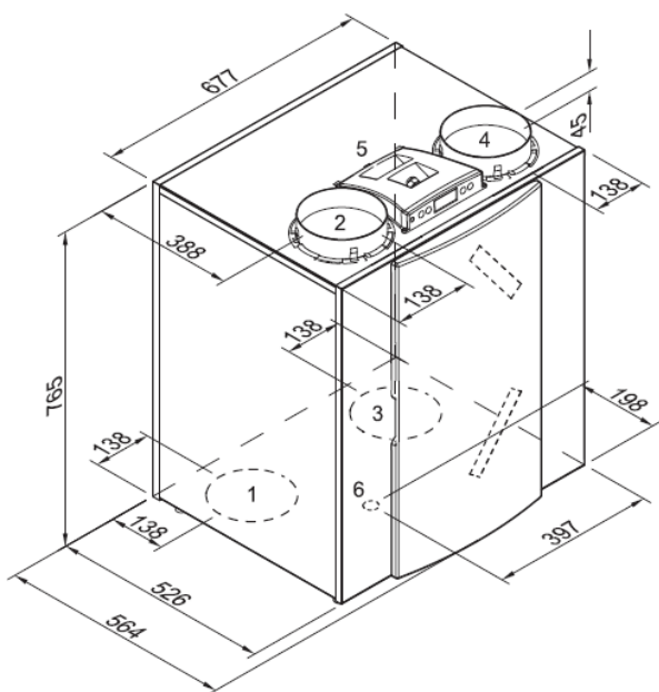
Rechtausführung 4/0
