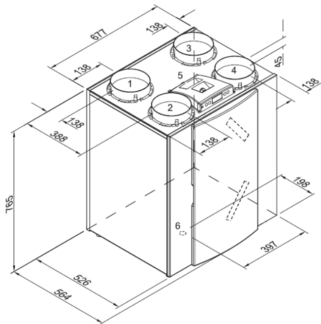
Rechtausführung 4/0
