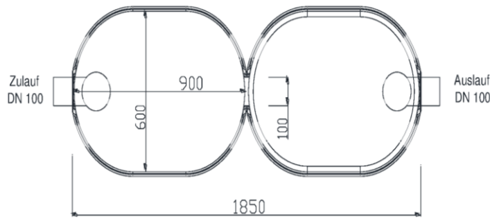
Schnitt D-D
