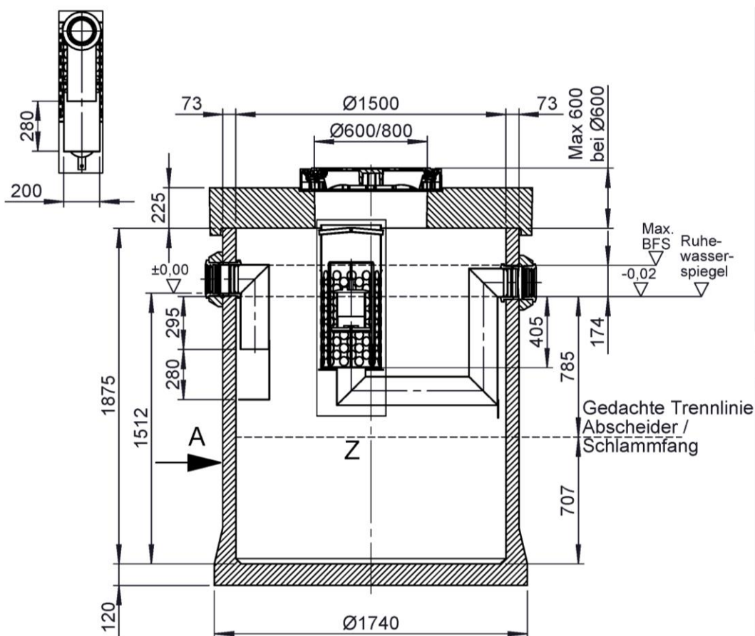
Ansicht A
