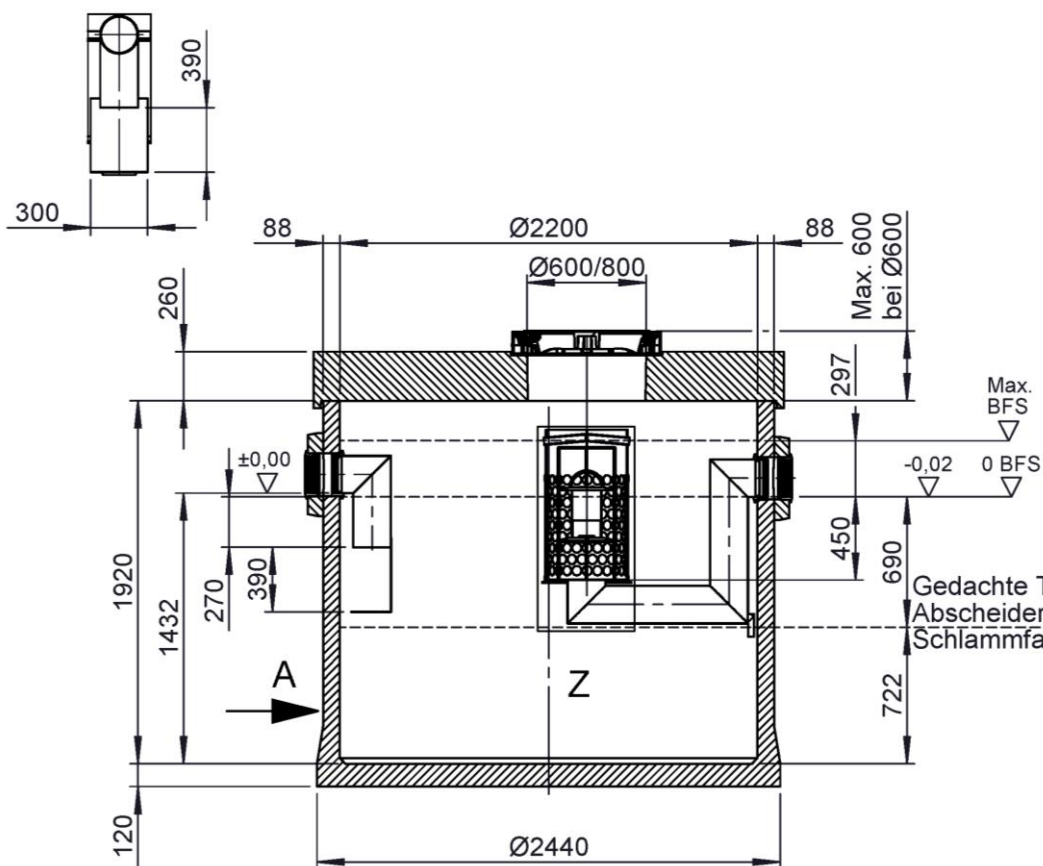
Ansicht A
