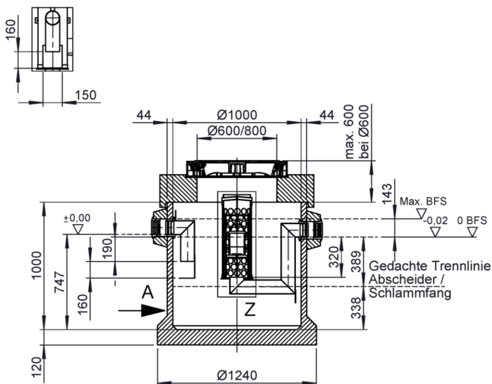
Ansicht A
