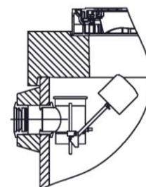
1601877 Zulaufausführung für Option Zulaufsperr (Zusatz verschlußseinrichtung)
