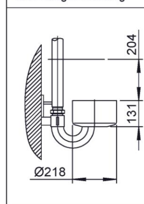
Ölabsaugvorrichtung
