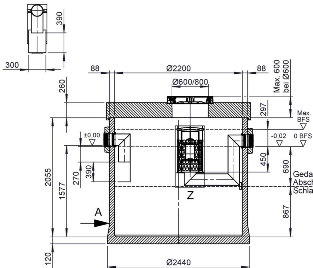
Ansicht A
