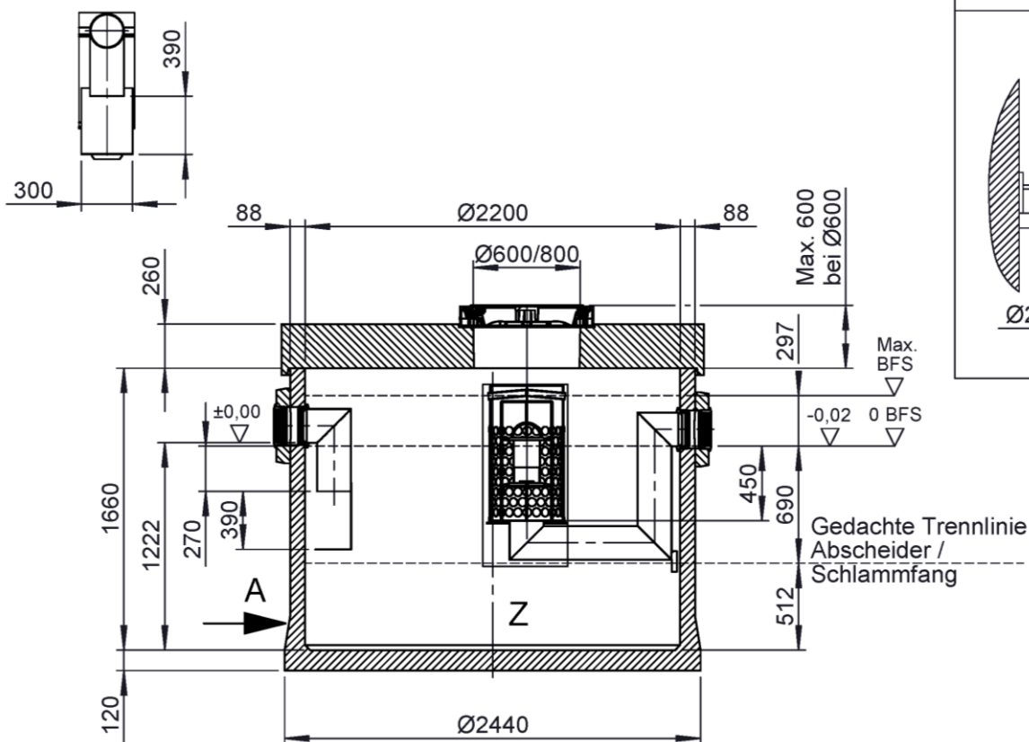
Ansicht A
