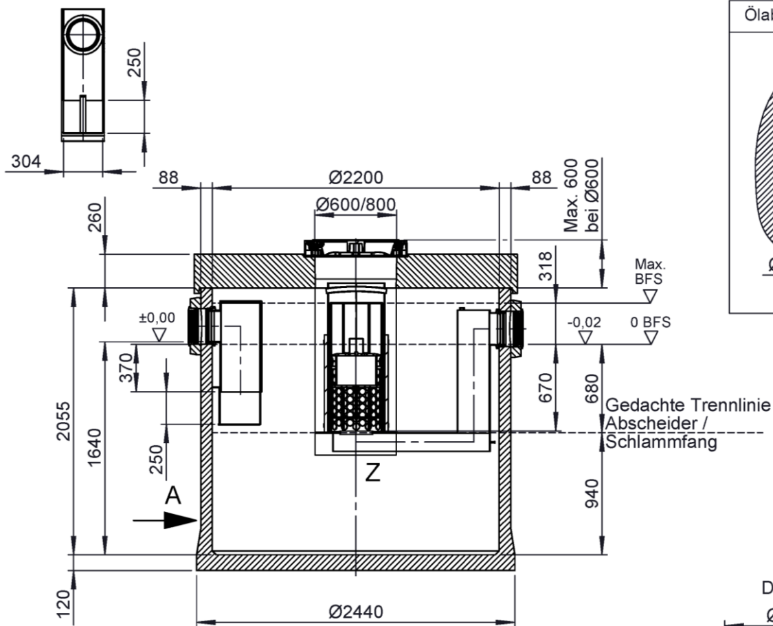
Ansicht A
