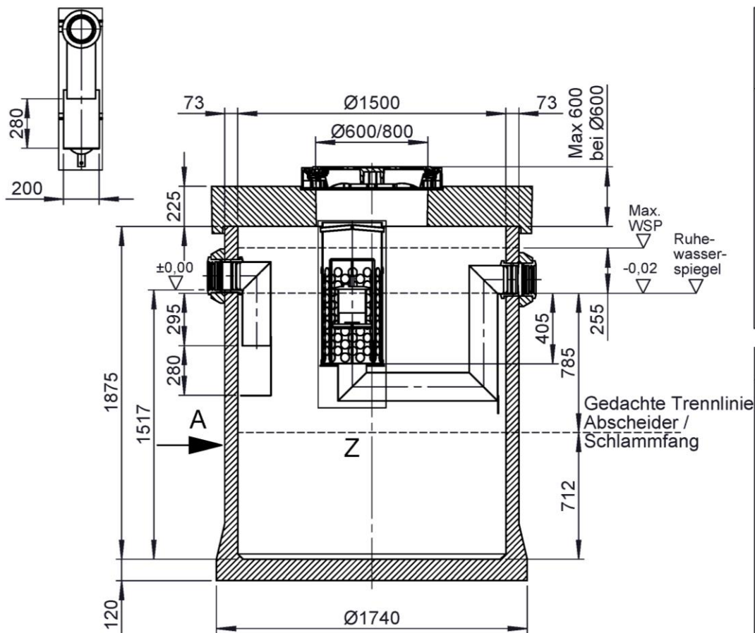
Ansicht A
