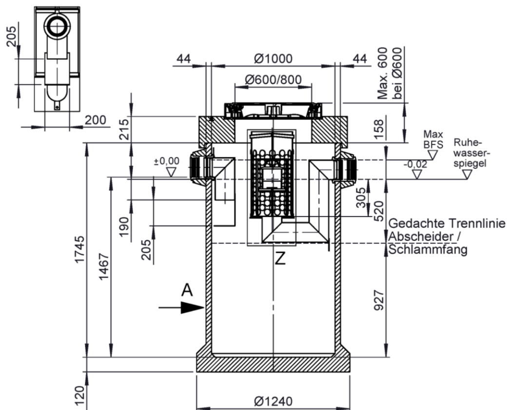
Ansicht A
