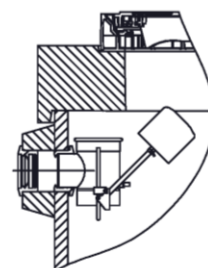
Ölabsaugvorrichtung
