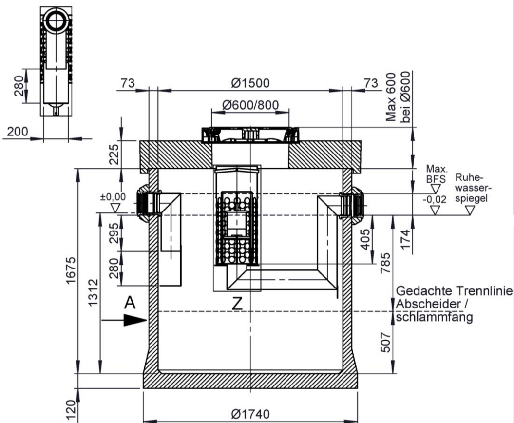
Ansicht A
