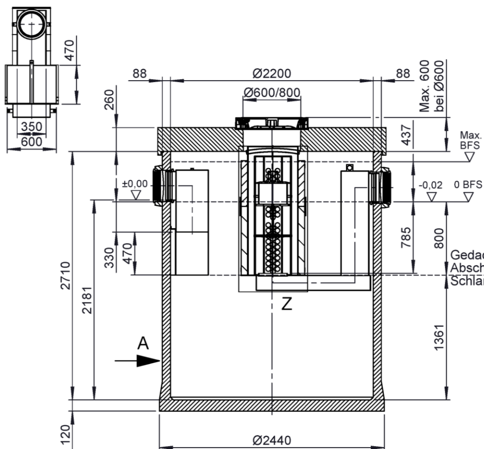
Ansicht A
