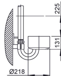
Ölabsaugvorrichtung
