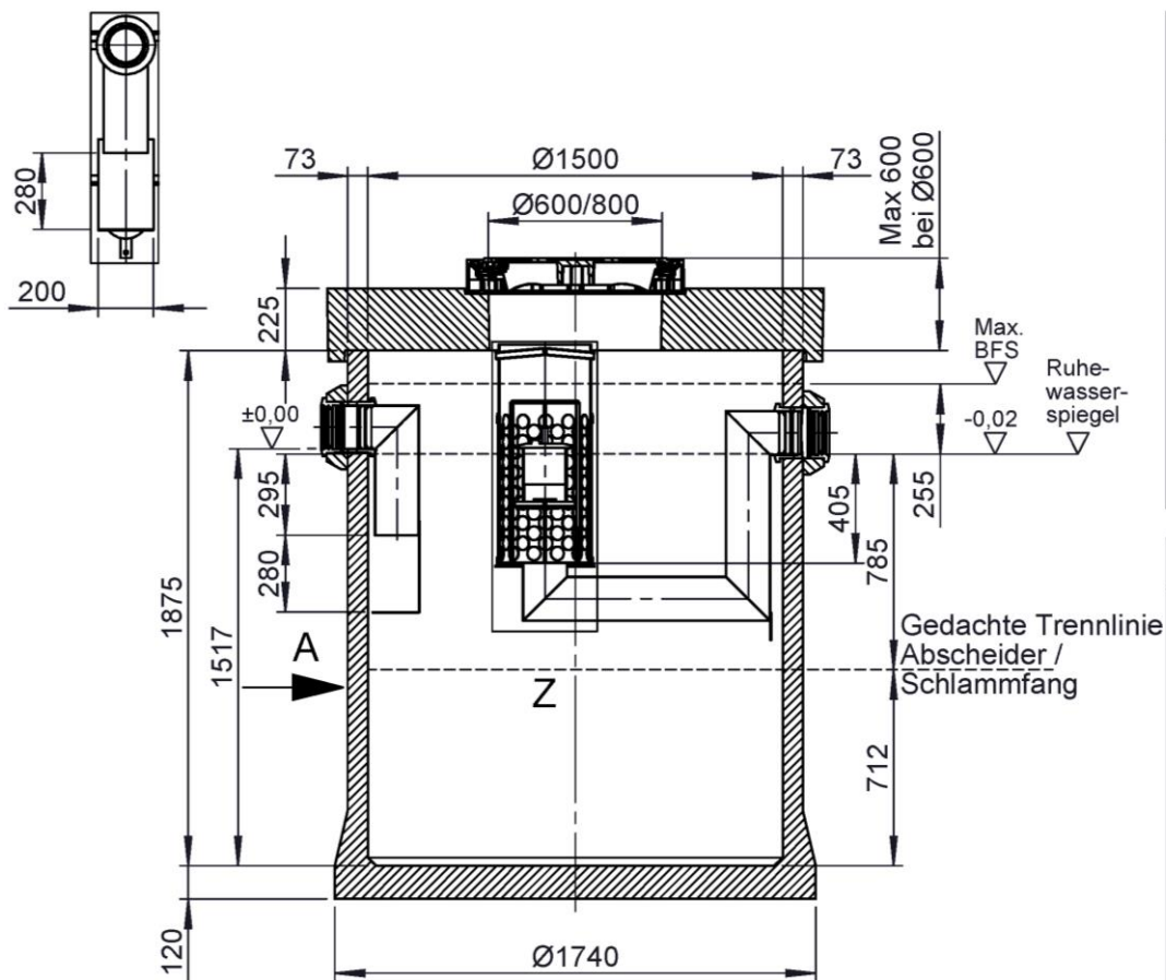
Ansicht A
