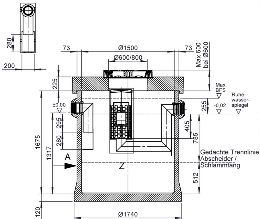
Ansicht A
