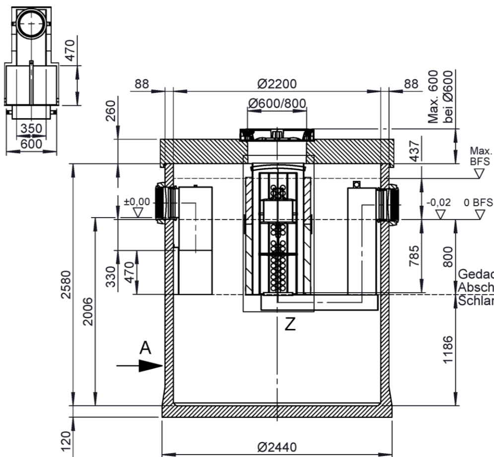
Ansicht A
