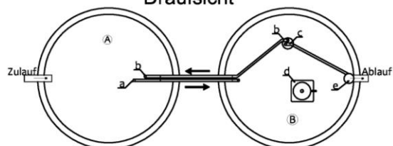
Draufsicht
