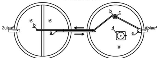
Draufsicht
