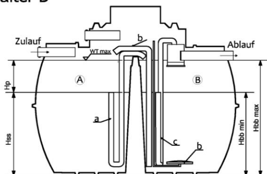
Behälter B
