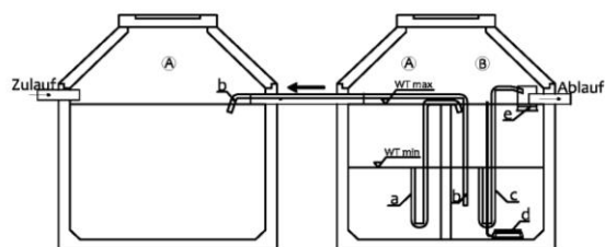
Seitenansicht
