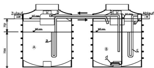
Seitenansicht
