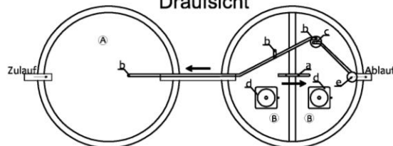
Draufsicht
