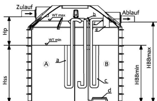
Seitenansicht
