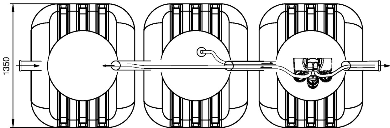
Grobfang/ Schlammsp.
