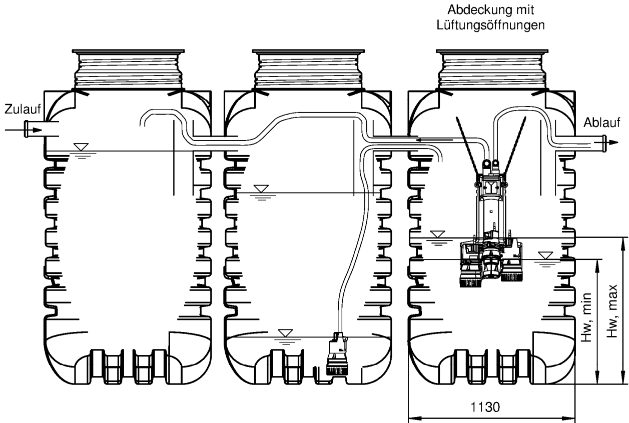
Grobfang/ Schlammsp.
