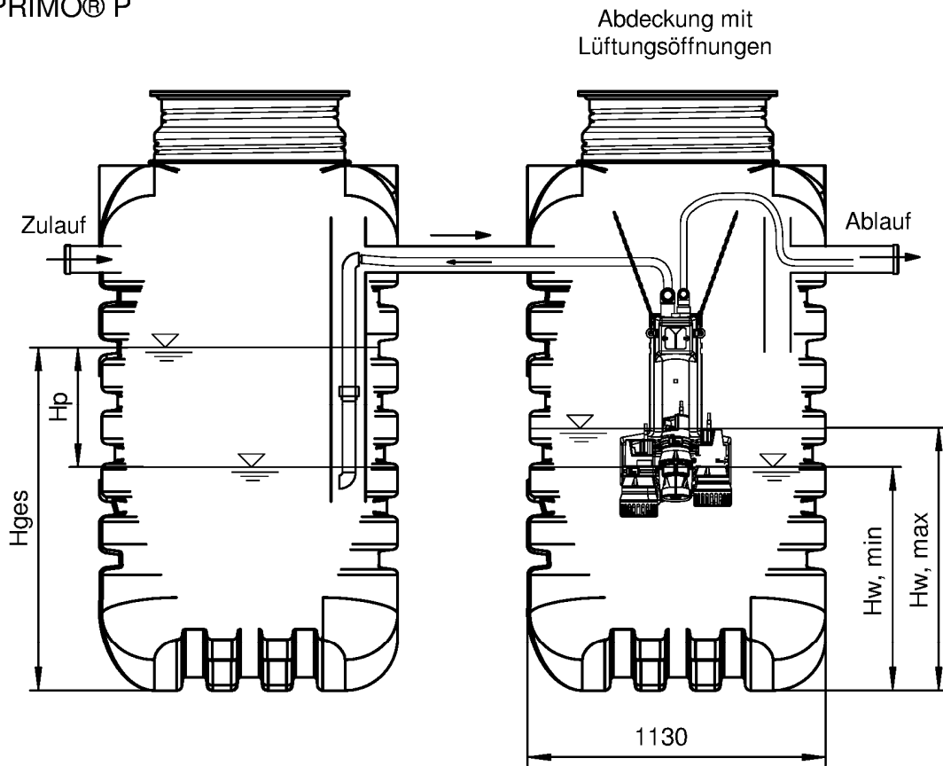
Grobfang/ Schlammsp.
