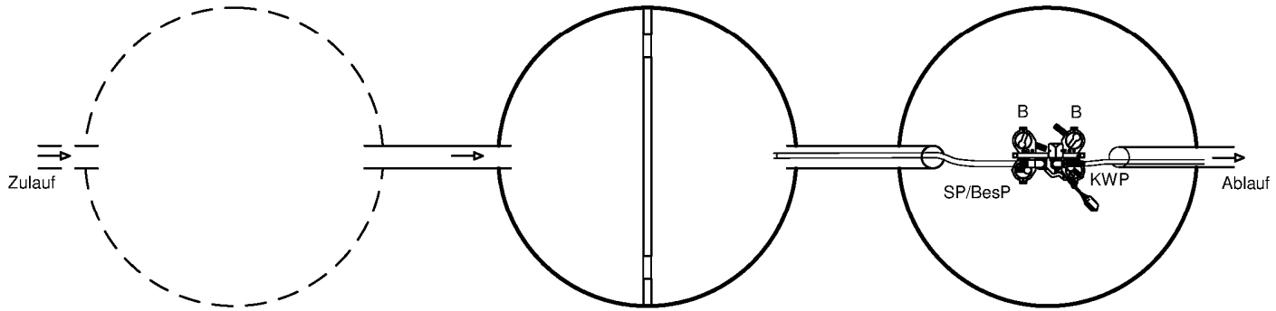
Grobfang Schlamm-speicher
